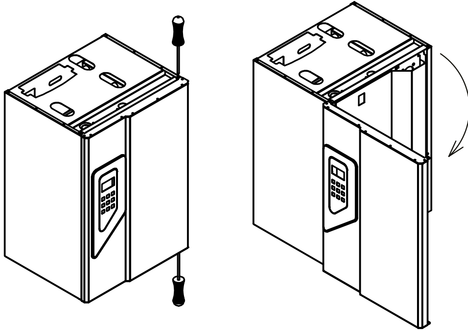
Kolay açılır kapanır kapak açma şekli ve yönü
